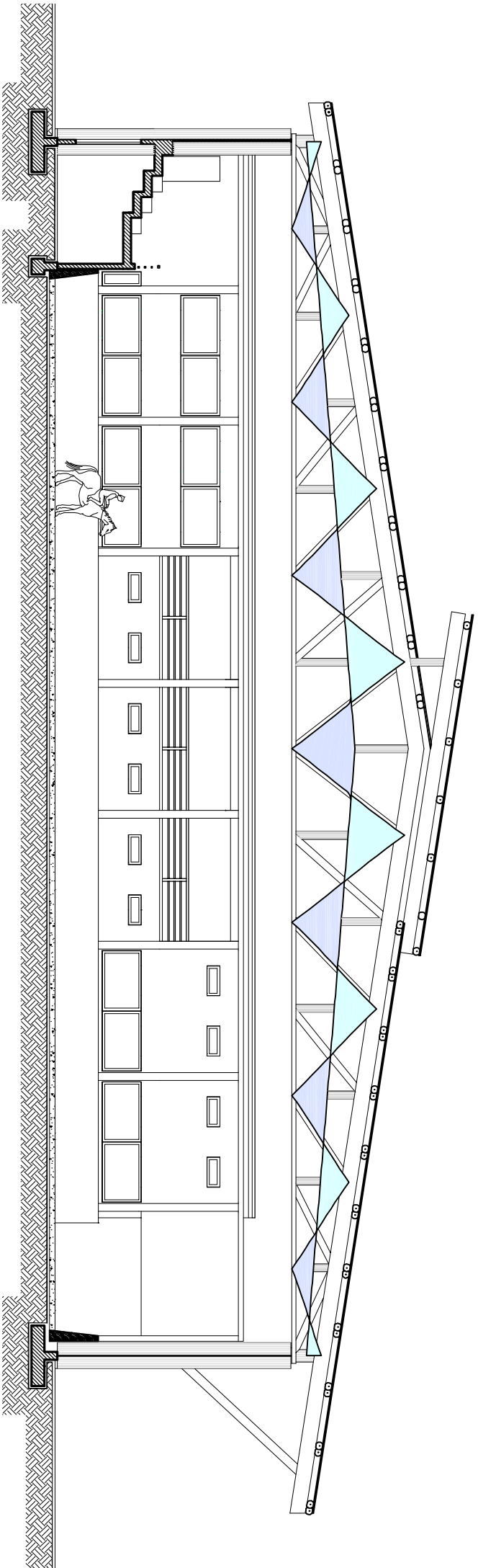
ESEMPIO DI CONTROSOFFITATURA TIPO "A ONDE" vista in sezione
