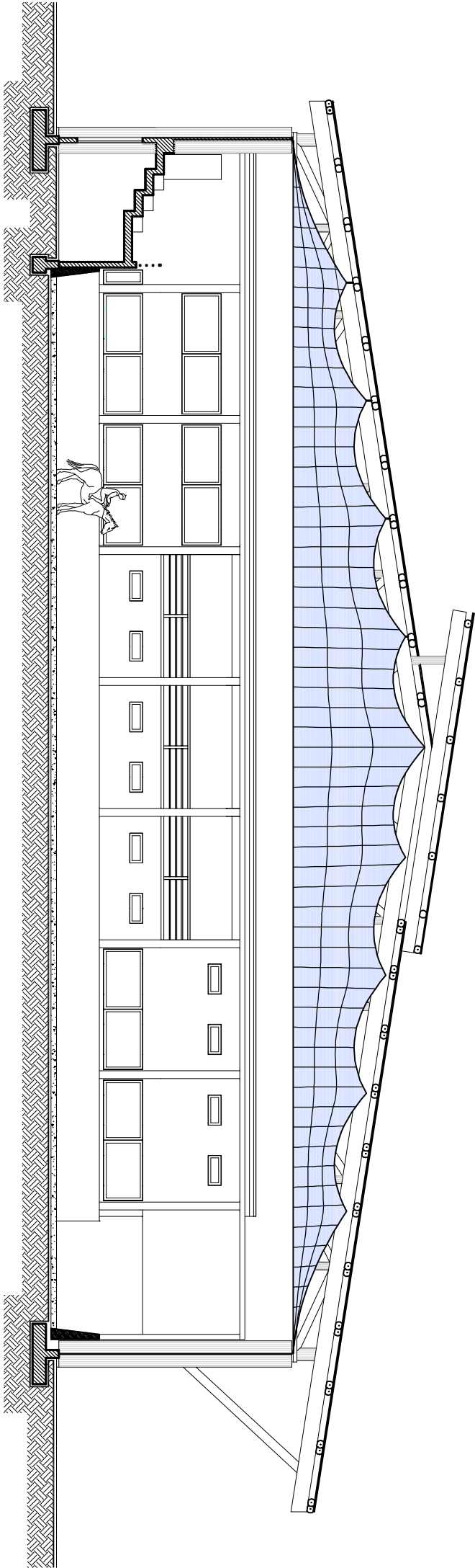
ESEMPIO DI CUNTIROSCUFFIATURA TIPO "A PUNTE" Vista in sezione
